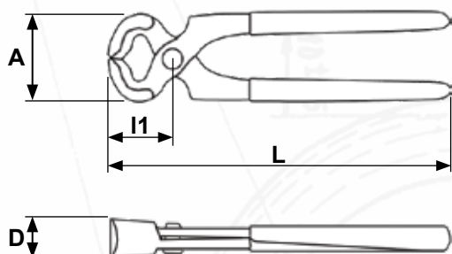
Kleště štípací čelní DIN ISO 5748 Carpenter's pincers DIN ISO 5748 Kneifzange DIN ISO 5748
