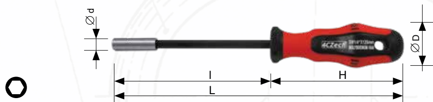
Držák bitů magnetický 1/4" s rukojetí profi Magnetic bit holder 1/4" with handle profi Bithalter magnetisch 1/4" mit Handgriff profi
