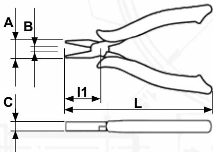
Kleště kombinované pro jemnou mechaniku Combination pliers for fine mechanics Kombizange für Feinmechanik
