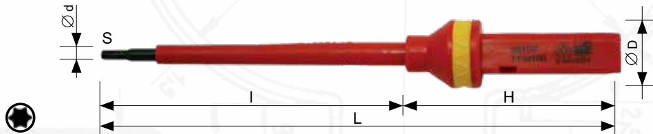
Šroubovák elektrikařský torx profil 1000V pro výměnnou rukojeť Insulated screwdriver torx tip profi for removable handle Elektriker-Schraubendreher torx profi 1000V für Wechselgriff
