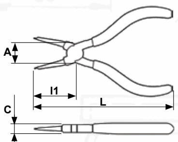
Kleště na pojistné kroužky pro otvory rovné DIN ISO 5256 Pliers for internal circlips straight DIN ISO 5256 Sicherungsringzange für Löcher gerade DIN ISO 5256
