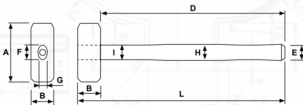
Palička s měkkými konci s dřevěnou rukojetí Double face soft hammer with wooden handle Schonhammer, rückschlagfrei, mit weichen Enden mit Holzgriff
