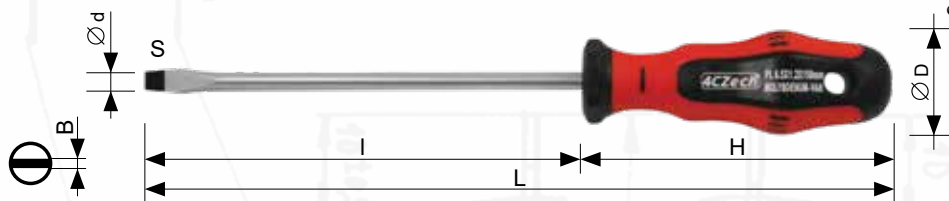
Šroubovák plochý profi Screwdriver flat tip profi Schraubendreher Schlitz profi
