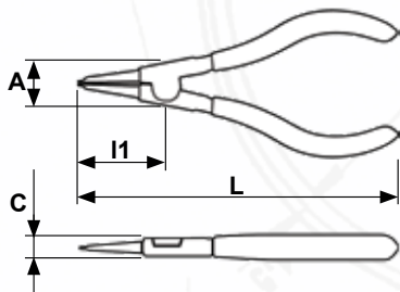
Kleště na pojistné kroužky pro hřídele vyhnuté 90° DIN ISO 5254 Pliers for external circlips bent 90° DIN ISO 5254 Sicherungsringzange für Wellen gekröpft 90° DIN ISO 5254
