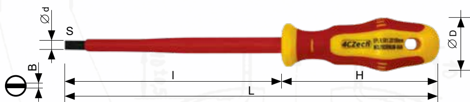
Šroubovák elektrikařský plochý profil 1000V Insulated screwdriver straight tip profil 1000V Elektriker-Schraubendreher Schlitz profil 1000V
