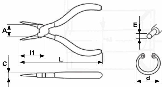
Kleště na pojistné kroužky pro otvory vyhnuté 90° DIN ISO 5256 Pliers for internal circlips bent 90° DIN ISO 5256 Sicherungsringzange für Löcher gekröpft 90° DIN ISO 5256
