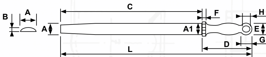
Pilník úsečový - tvar PZP File halfround - shape PZP Feile halbrund - Form PZP
