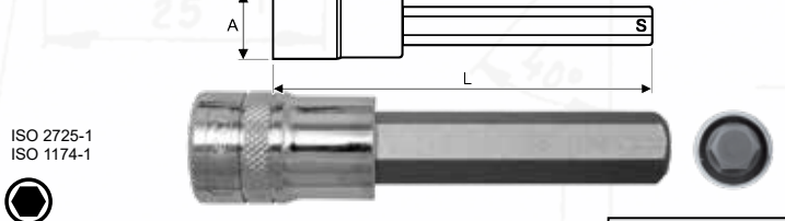
ISO 2725-1 ISO 1174-1 1/2" Zástrčná hlavice imbus prodloužená 1/2" HEX Bit socket long-reach type 1/2" Steckschlüssel-Einsatz imbus verlängert
