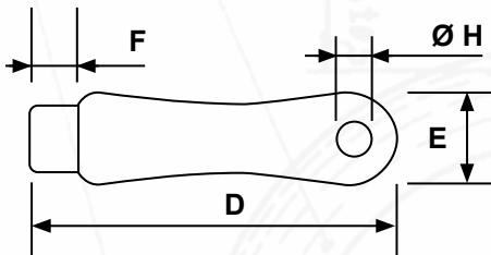
Násada na pilník a rašple dřevěná File and rasp handle wooden Feilen- und Raspelgriff aus Holz
