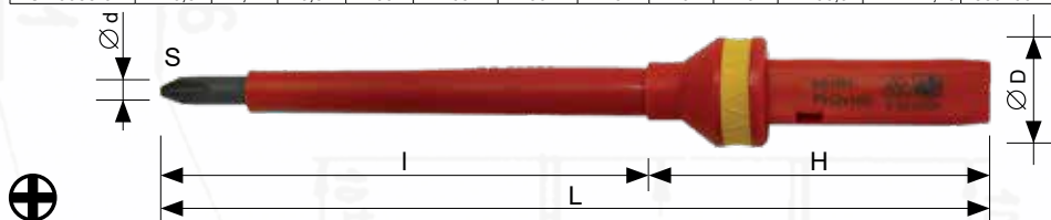
Šroubovák elektrikařský phillips profil 1000V pro výměnnou rukojeť Insulated screwdriver phillips tip profi for removable handle Elektriker-Schraubendreher Phillips profi 1000V für Wechselgriff
