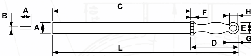
Pilník plochý lehký - tvar PLO File hand thin - shape PLO Feile flachstumpf - Form PLO
