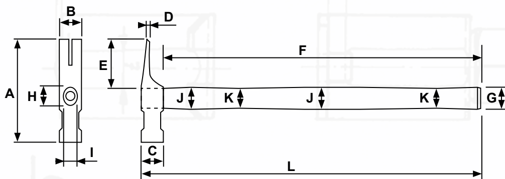
Kladivo tesařské s rovnými čelistmi Carpenter's hammer with straight jaws Zimmermannshammer mit geraden Backen
