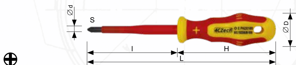
Šroubovák elektrikařský phillips profil 1000V Insulated screwdriver phillips tip profil 1000V Elektriker-Schraubendreher Phillips profil 1000V
