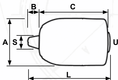
Skličidlo vrtačkové rychloupínací, plastové, se závitem Drill chuck self-tightening, plastic, with thread Bohrfutter mit Radialverriegelung Kunststoffausführung, mit Gewinde
