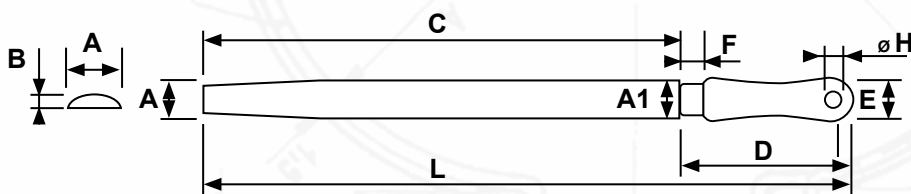
Rašple úsečová strojní sek PRP Halfround rasp machine cut PRP Halbrundraspel Maschinenhieb PRP
