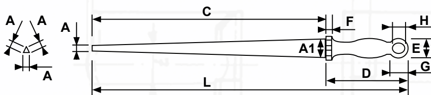
Pilník tříhranný - tvar PZT File three-square - shape PZT Feile dreikant - Form PZT
