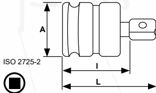
ISO 2725-2 1/2" Univerzální kardan průmyslový CrMo + trn, o-kroužek 1/2" Impact universal joint CrMo + pin, o-ring - 1/2" Schlag Universal-Kardangelenk CrMo + Dorn, O-Ring
