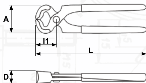
Kleště štípací čelní precizní DIN ISO 5748 End cutting nippers DIN ISO 5748 Präzisions-Kneifzange DIN ISO 5748
