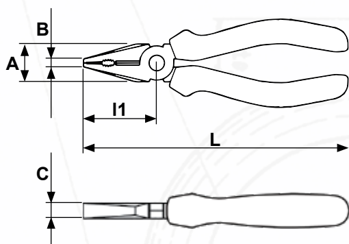
Kleště kombinované DIN ISO 5746 All purpose pliers DIN ISO 5746 Kombizange DIN ISO 5746
