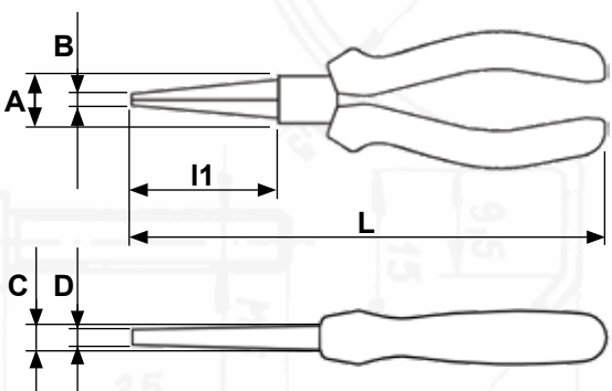
Kleště na drát s plochými čelistmi DIN ISO 5745 Flat nose pliers DIN ISO 5745 Verdrahtungszange mit flachen Backen DIN ISO 5745
