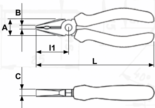
Kleště kombinované DIN ISO 5746 s funkcí krimpování koncovek Combination pliers DIN ISO 5746 with end crimping function Kombizange DIN ISO 5746 mit Funktion Crimpen von Klemmen
