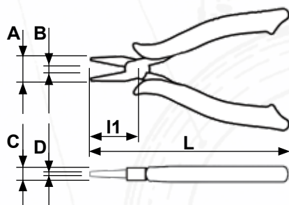
Kleště na drát s kulatými čelistmi pro jemnou mechaniku Round nose pliers for fine mechanics Verdrahtungszeuge mit runden Backen für die Feinmechanik
