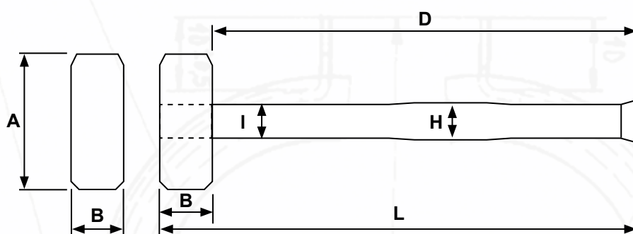
Palička bezodskoková s plastovou rukojetí Dead blow hammer with plastic handle Schonhammer, rückschlagfrei mit Kunststoffgriff
