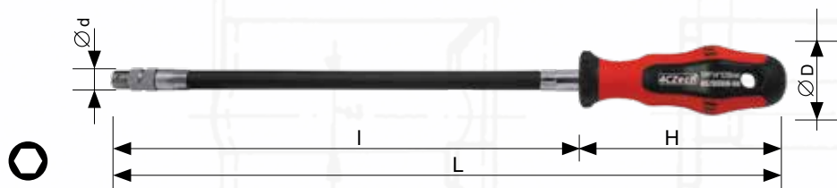
Držák bitů 1/4" FLEXI s rukojetí profi Flexible driver 1/4" with handle profi Bithalter FLEXI 1/4" mit Handgriff profi
