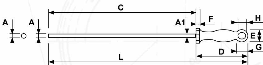
Pilník kruhový - tvar PZK File round - shape PZK Feile rund - Form PZK
