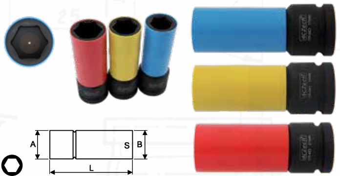
1/2" hlavice nástrčná, na ALU disky kol, délka 85 mm 1/2" deep impact socket, for aluminium wheel discs, length 85 mm 1/2" Steckschlüssel, für Alu-Radscheiben, Länge 85 mm
