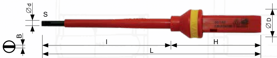
Šroubovák elektrikařský plochý profil 1000V pro výměnnou rukojeť Insulated screwdriver straight tip profi for removable handle Elektriker-Schraubendreher Schlitz profi 1000V für Wechselgriff
