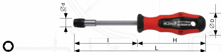
Držák bitů 1/4" s rukojetí s pojistkou profi Quick release 1/4" with handle profi Bithalter 1/4" mit Handgriff mit Sicherung profi
