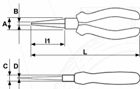
Kleště na drát s kulatými čelistmi DIN ISO 5745 Round nose pliers DIN ISO 5745 Verdrahtungszange mit runden Backen DIN ISO 5745
