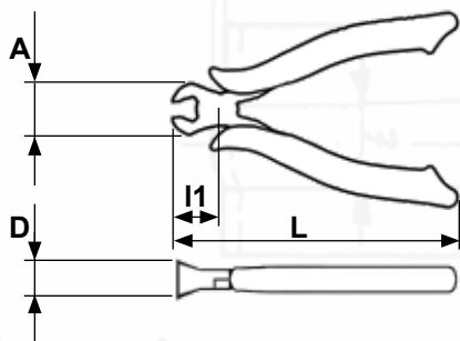
Kleště štípací čelní pro jemnou mechaniku End cutting pliers for fine mechanics Kneifzange für die Feinmechanik
