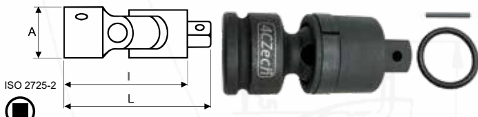
ISO 2725-2 3/4" Univerzální kardan průmyslový CrMo + trn, o-kroužek 3/4" Impact universal joint CrMo + pin, o-ring 3/4" Schlag Universal-Kardangelenk CrMo + Dorn, O-Ring
