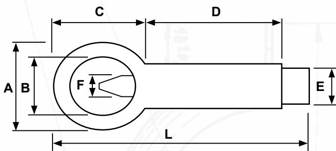
Trháč matic mechanický Mechanical nut splitter Mechanischer Mutternsprenger
