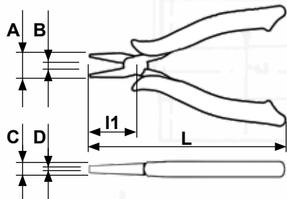
Kleště na drát s půlkulatými čelistmi pro jemnou mechaniku Long nose pliers for fine mechanics
