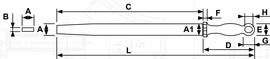
Pilník dílenský plochošpičatý PZA Engineer's file flat PZA Werkstattfeile flachspitz PZA
