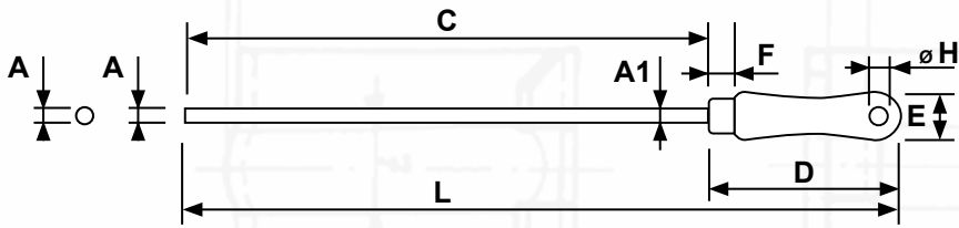
Rašple kruhová strojní sek 6 PRK Round rasp machine cut 6 PRK Rundraspel Maschinenhieb 6 PRK
