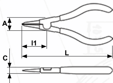
Kleště na pojistné kroužky pro hřídele rovné DIN ISO 5254 Pliers for external circlips straight DIN ISO 5254 Sicherungsringzange für Wellen gerade DIN ISO 5254
