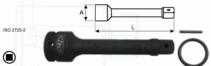
ISO 2725-2 3/4" Nástavec průmyslový CrMo + trn, o-kroužek 3/4" Impact Extension bar CrMo + pin, o-ring 3/4" Schlag-Verlängerung CrMo + Dorn, O-Ring
