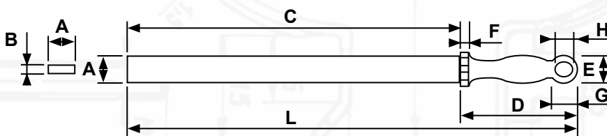
Pilník plochý silný - tvar PSO File hand - shape PSO Feile flachstumpf - Form PSO
