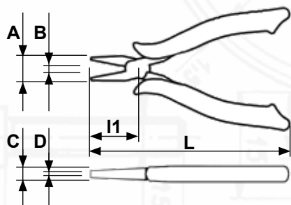
Kleště na drát s půlkulatými jehlovými čelistmi pro jemnou mechaniku Needle nose pliers for fine mechanics
