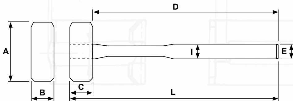
Palička s plastovou rukojetí Mallet with plastic handle Fäustel mit Kunststoffgriff
