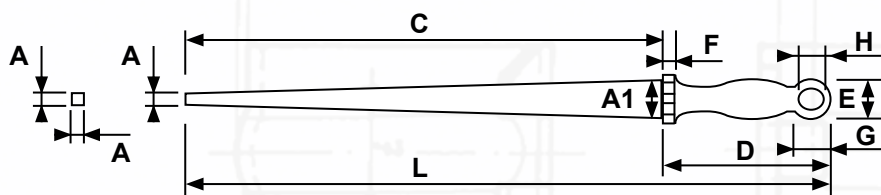
Pilník čtyřhranný - tvar PZC File square - shape PZC Feile vierkant - Form PZC
