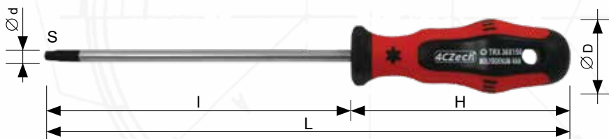
Šroubovák torx profi Screwdriver torx tip profi Schraubendreher Torx profi
