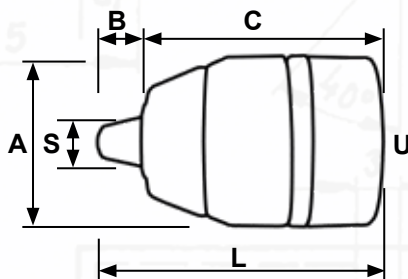
Skličidlo vrtačkové rychloupínací, kovové Lock HM, se závitem Drill chuck self-tightening, metal Lock HM, with thread Bohrfutter mit Radialverriegelung Metallausführung, mit Gewinde
